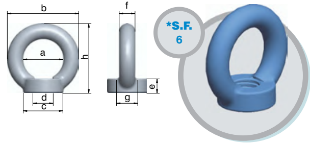
GOLFARE FEMMINA DIN 582 - LIFTING EYE NUT DIN 582
